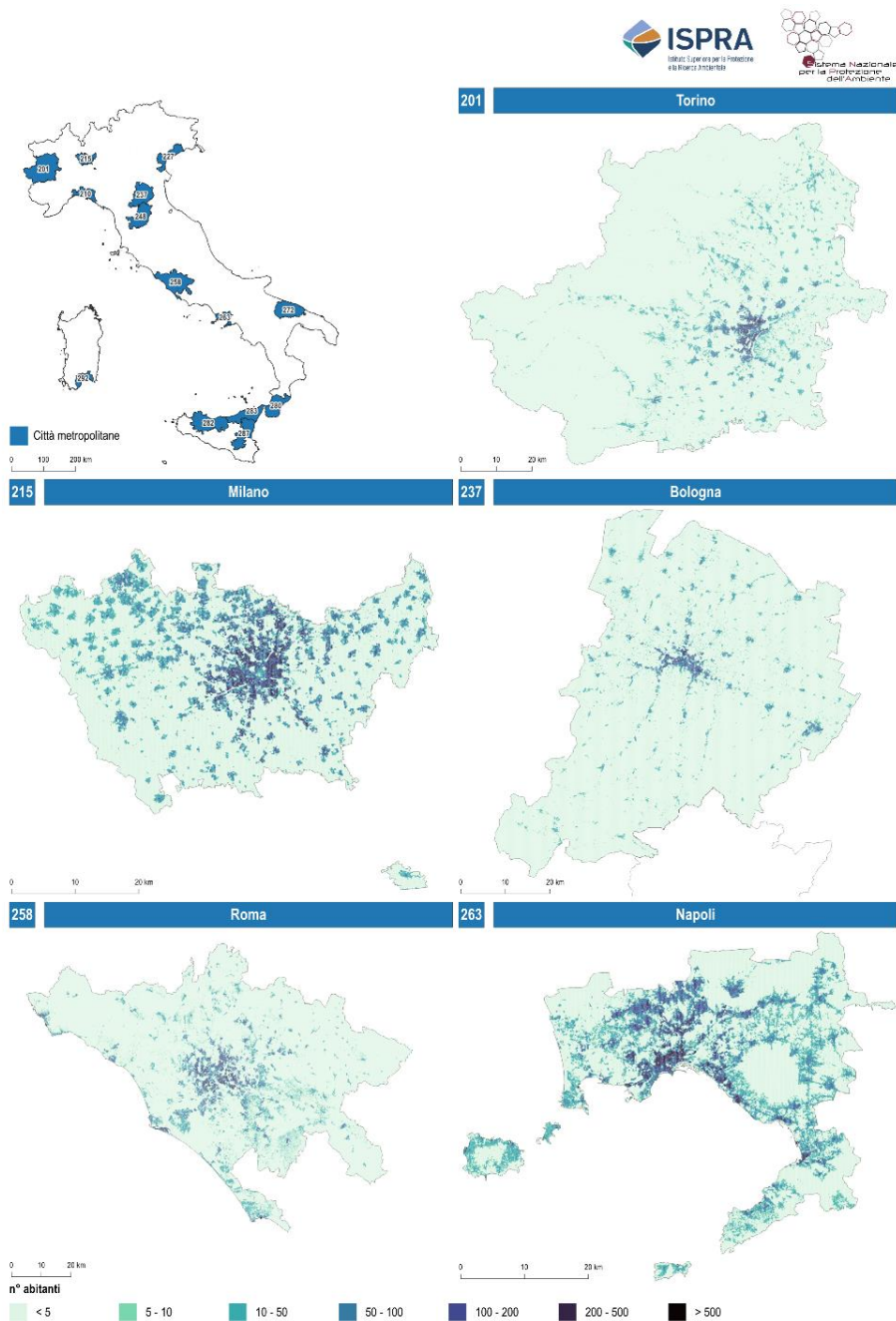
Figura 53. Esempio di spazializzazione del dato di popolazione Istat (relativo alle sezioni di censimento per il 2021) per 5 città metropolitane. Il dato è stato realizzato anche per la restante parte del territorio nazionale. Fonte: elaborazioni ISPRA su cartografia SNPA, dati Istat, CLMS e OSM
