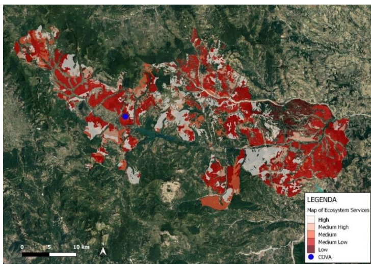
Figura 156. Mappa rappresentativa dell'idoneità rispetto ai Servizi Ecosistemici
